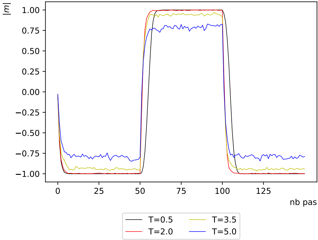
Aimantation en présence d'un champ magnétique variant de h=-2.5 à +2.5 , N=32, k=50
